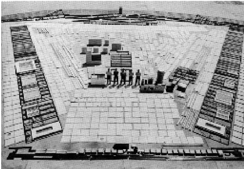
Figure 1.23: Building components of the Lustron-house (tussen traditie en experiment: De wonderlijke wereld van de woning Jan Westra 1990)
